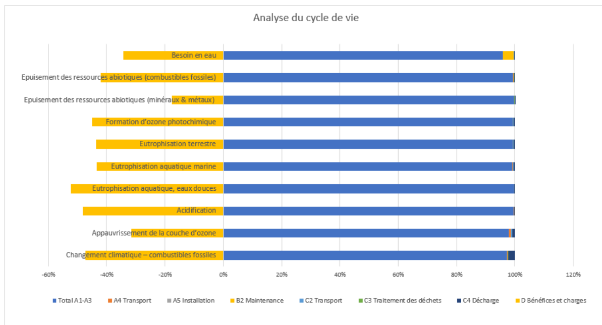
Figure 1 : Impacts environnementaux des portes d'entrée D72_D.1.21 tout au long de son cycle de vie (impacts des modules de production A1-A3 = 100 %)
