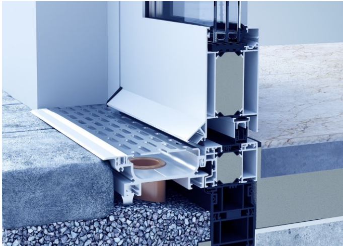
[Foto: heroal D 72 Null-Barriere mit Drainagesystem]
