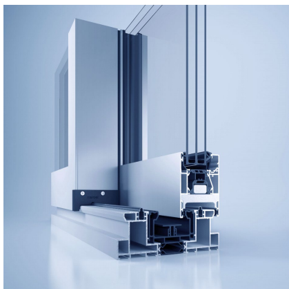
[heroal S 65]
